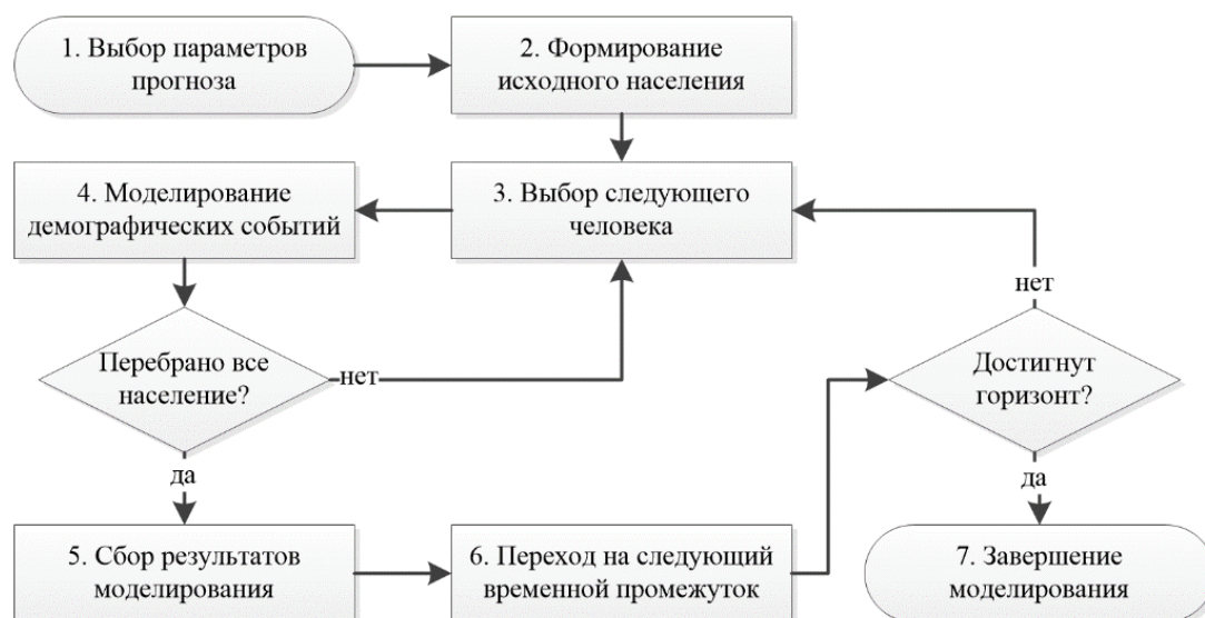
Рис. 1. Алгоритм прогнозирования
